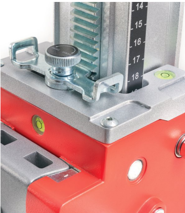
Doppia livella e leva per arresto calata
